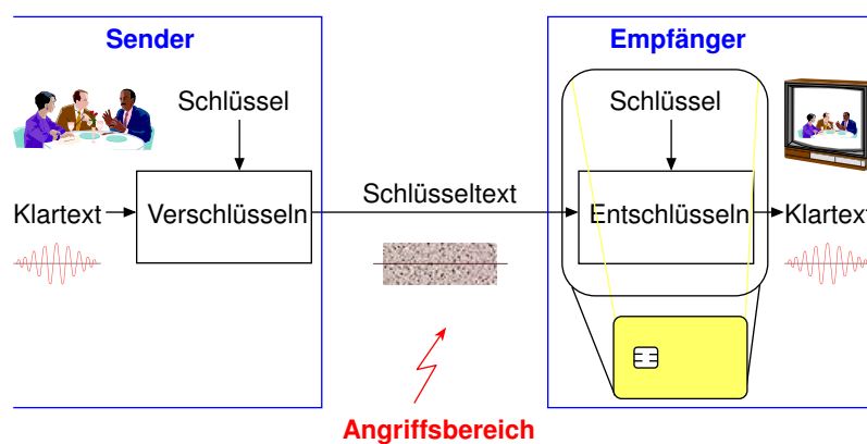
Abbildung 2.3: Verschlüsselung auf Übertragungswegen
